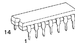
P (DIP14-P-300-2.54) Weight : 0.96g (Typ.)
