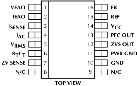
ML4822 16-Pin SOIC (S16W)
