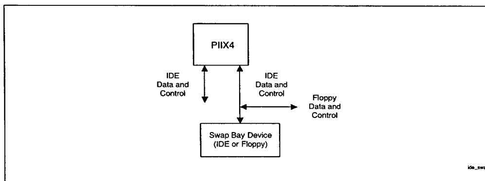
Figure 6. PIIX4 IDE Swap Bay Example
